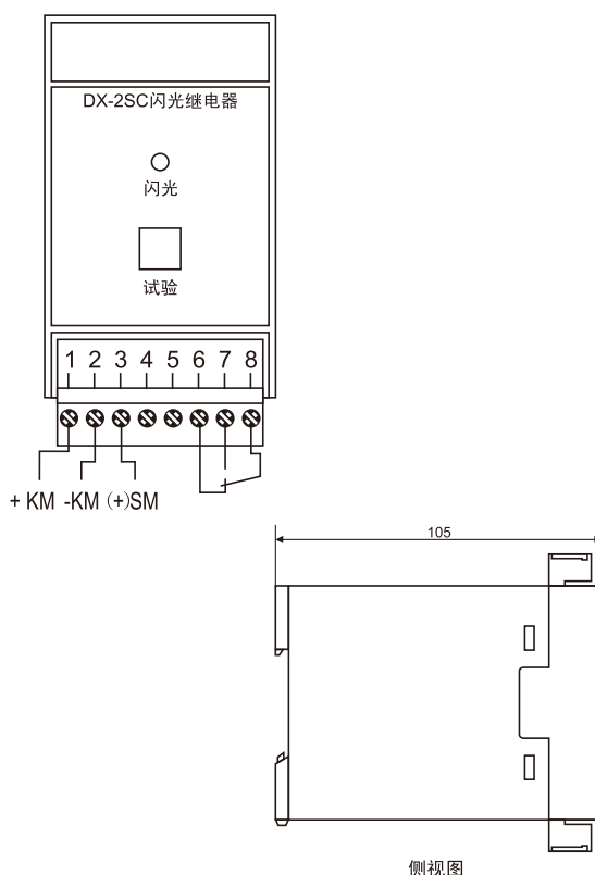
侧视图
